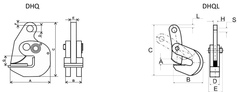
Рисунок 1. Размеры захвата
