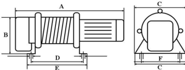
Рисунок 1. Габаритные размеры.
